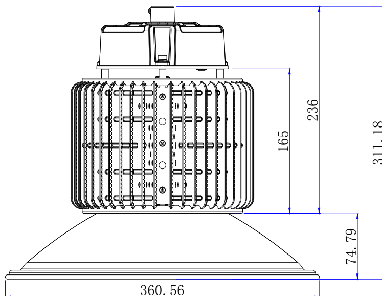
100° Reflector
